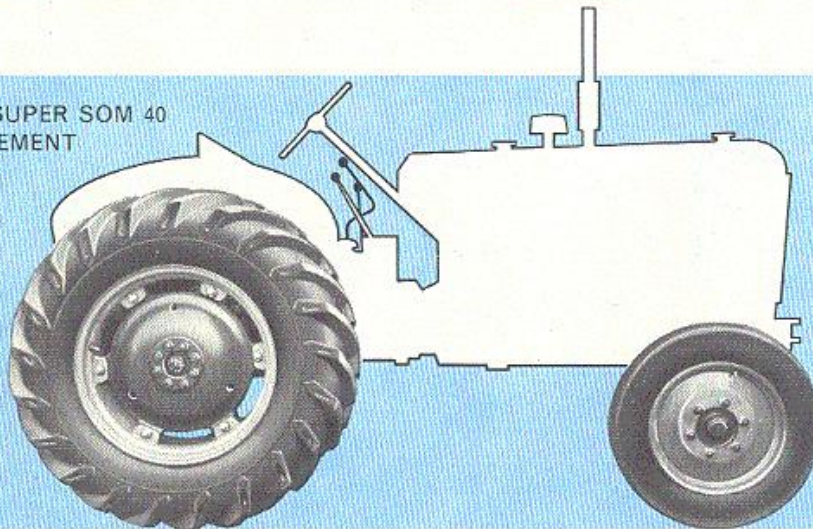
SUR ROUES ARRIERE 1, 2 OU 3 MASSES DE 50 kg PAR ROUE
